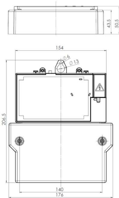
DD3 mit Klemmendeckel 60 mm
