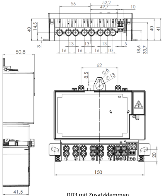
DD3 mit Zusatzklemmen
