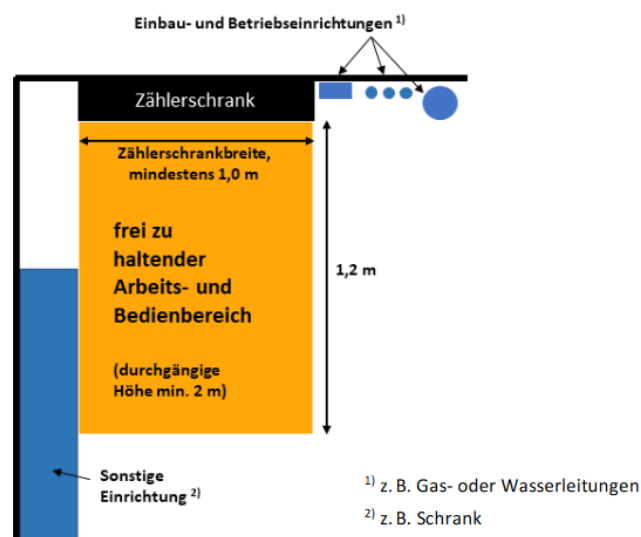
Abbildung 3 - Arbeits- und Bedienbereich vor dem Zählerschrank
